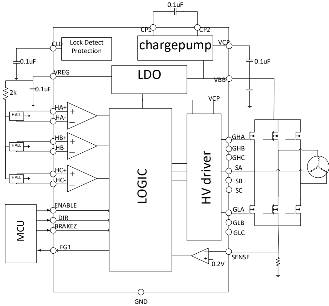
图 4 GC4938 典型应用图
