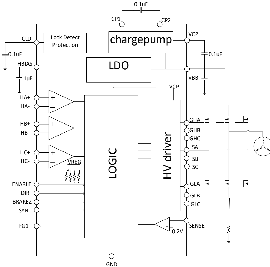
图 1 GC4938 内部框图
