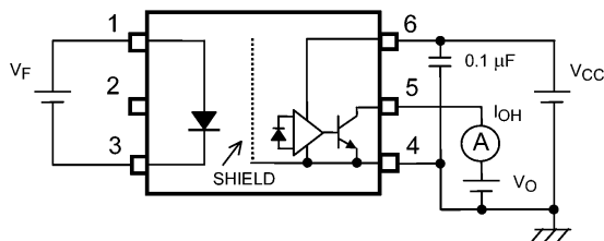
Fig. 13.1.1 I_{OH} Test Circuit
