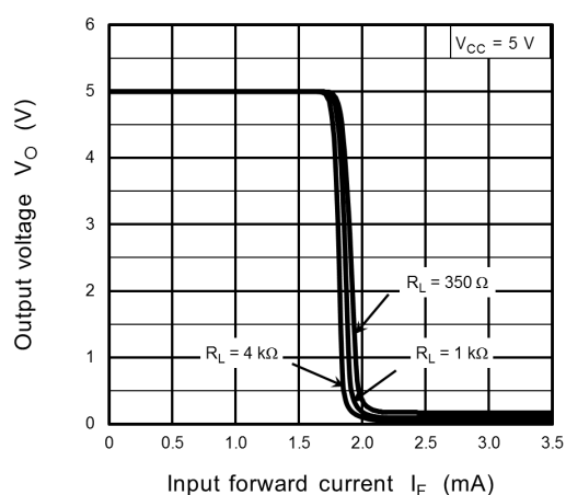
Fig. 13.2.5 V_O - I_F
