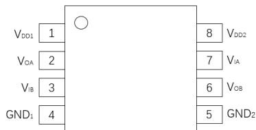
图 5. Pai122E6x 管脚定义
