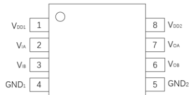
图 3. Pai120E6x 管脚定义
