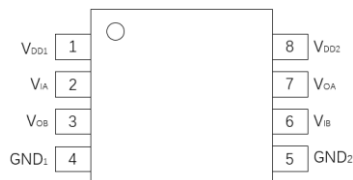
图 4. Pai121E6x 管脚定义
