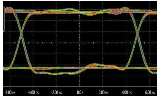
图 11. Pai12xExx 眼图
