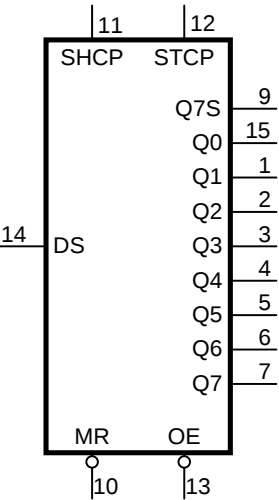
图 1 逻辑符号
