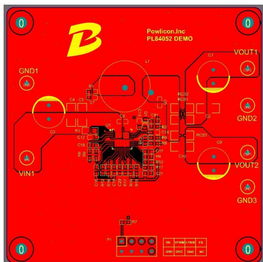
Fig. 5 Top lay
