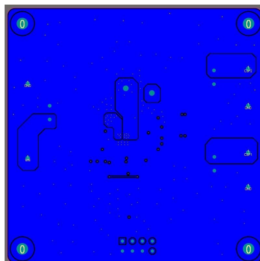
Fig. 6 Bottom lay
