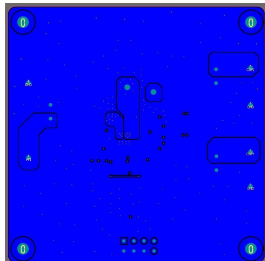
Fig. 5 Bottom lay
