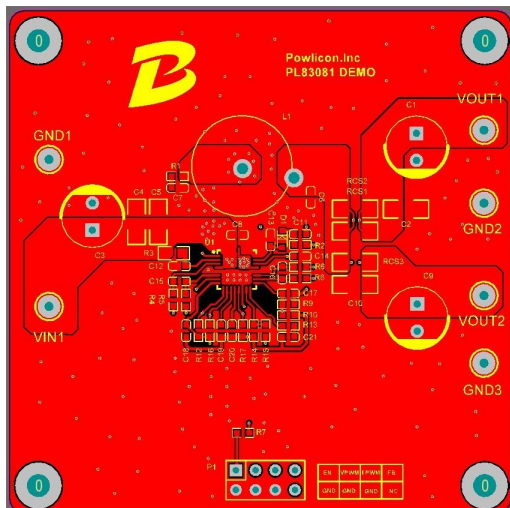
Fig. 4 Top lay
