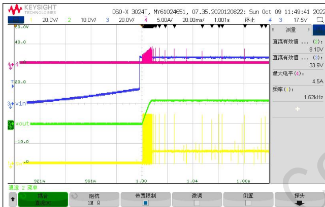
Fig. 4 VIN Start-up IOUT=0A
