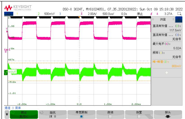
Fig. 17 Load Transient IOUT=2-5A I-ramp=1A/us
