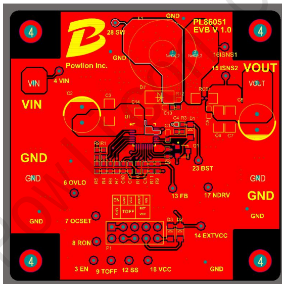
Fig. 24 Top lay
