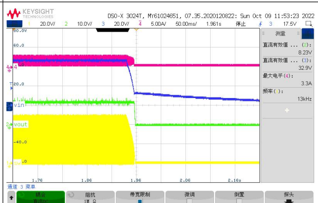
Fig. 7 VIN Shutdown IOUT=1A
