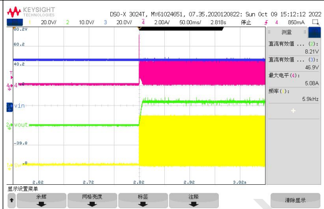
Fig. 9 EN Start-up IOUT=1A
