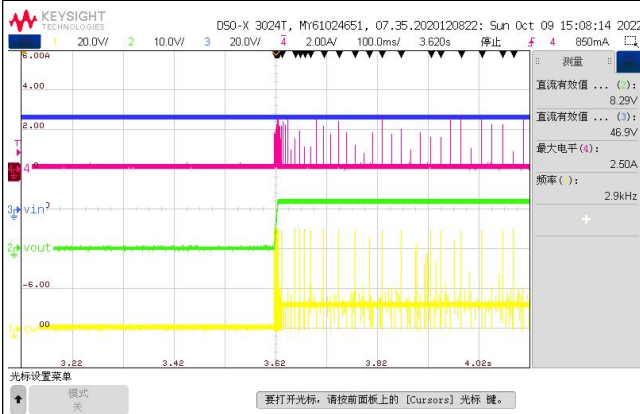
Fig. 8 EN Start-up IOUT=0A
