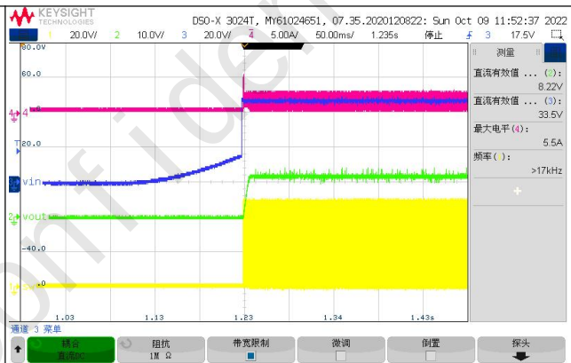
Fig. 5 VIN Start-up IOUT=1A
