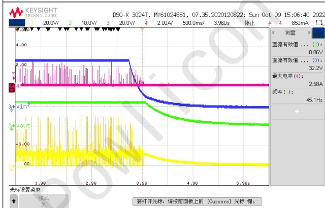
Fig. 6 VIN Shutdown IOUT=0A
