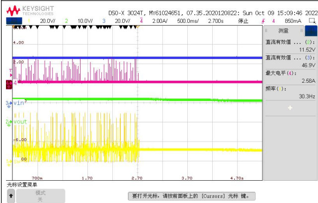
Fig. 10 EN Shutdown IOUT=0A
