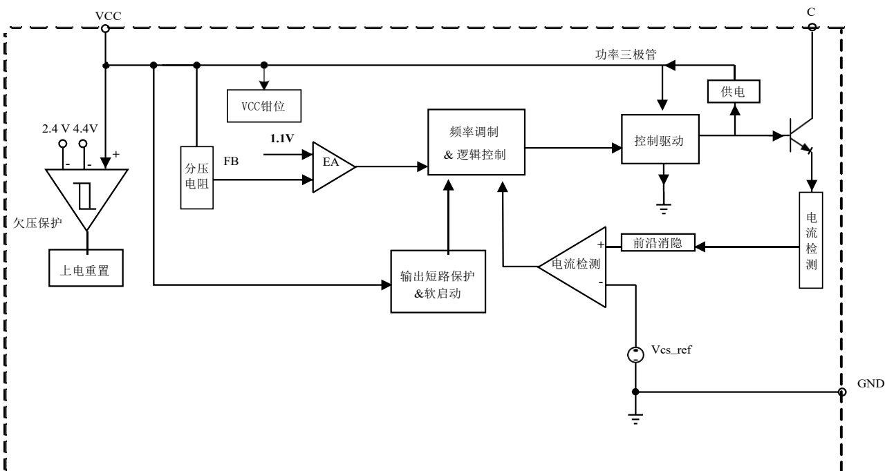
图 4 ICW4008 内部框图
