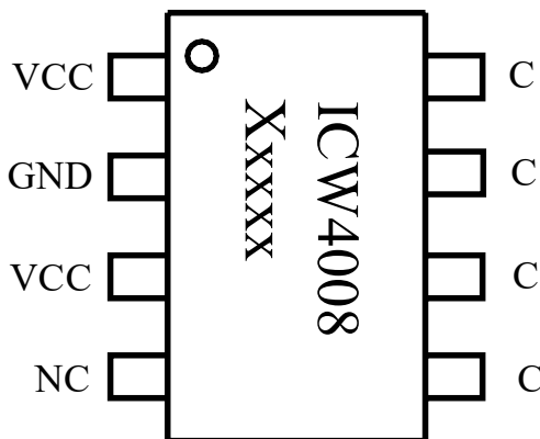
图 3 管脚封装图
