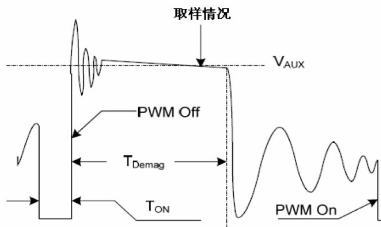
图4 辅助绕组电压波形图
