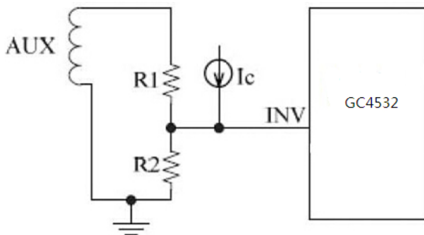
图5 线损补偿电路
