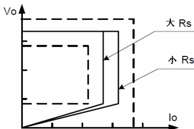
图3 输出功率随 R_S 变化曲线
