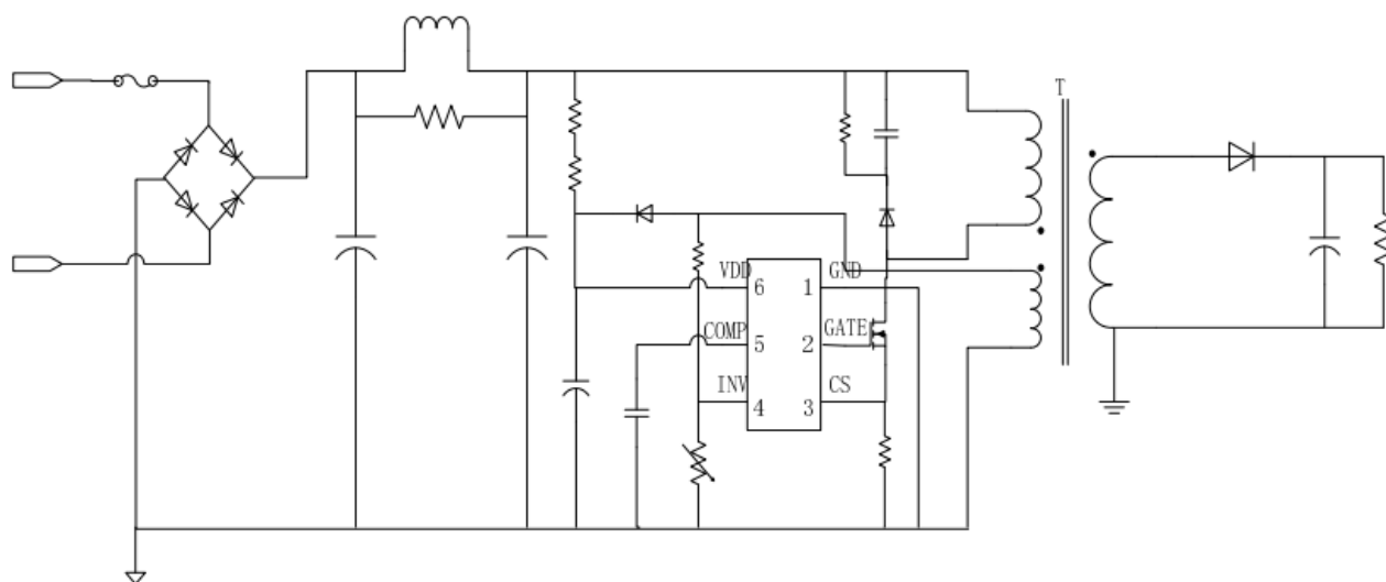
GC4532 典型应用电路图
