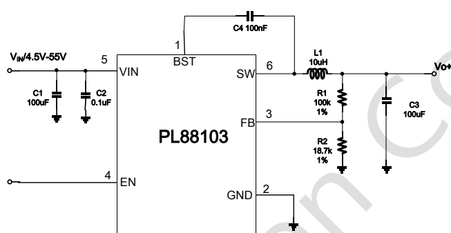
Fig. 1 Schematic
