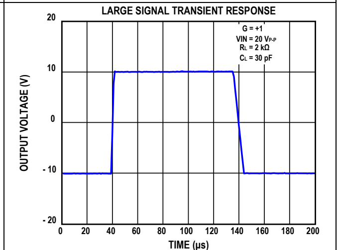
图16. 大信号瞬变响应
