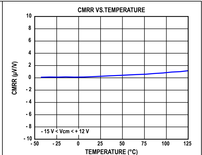
图14. 共模抑制比与温度的关系
