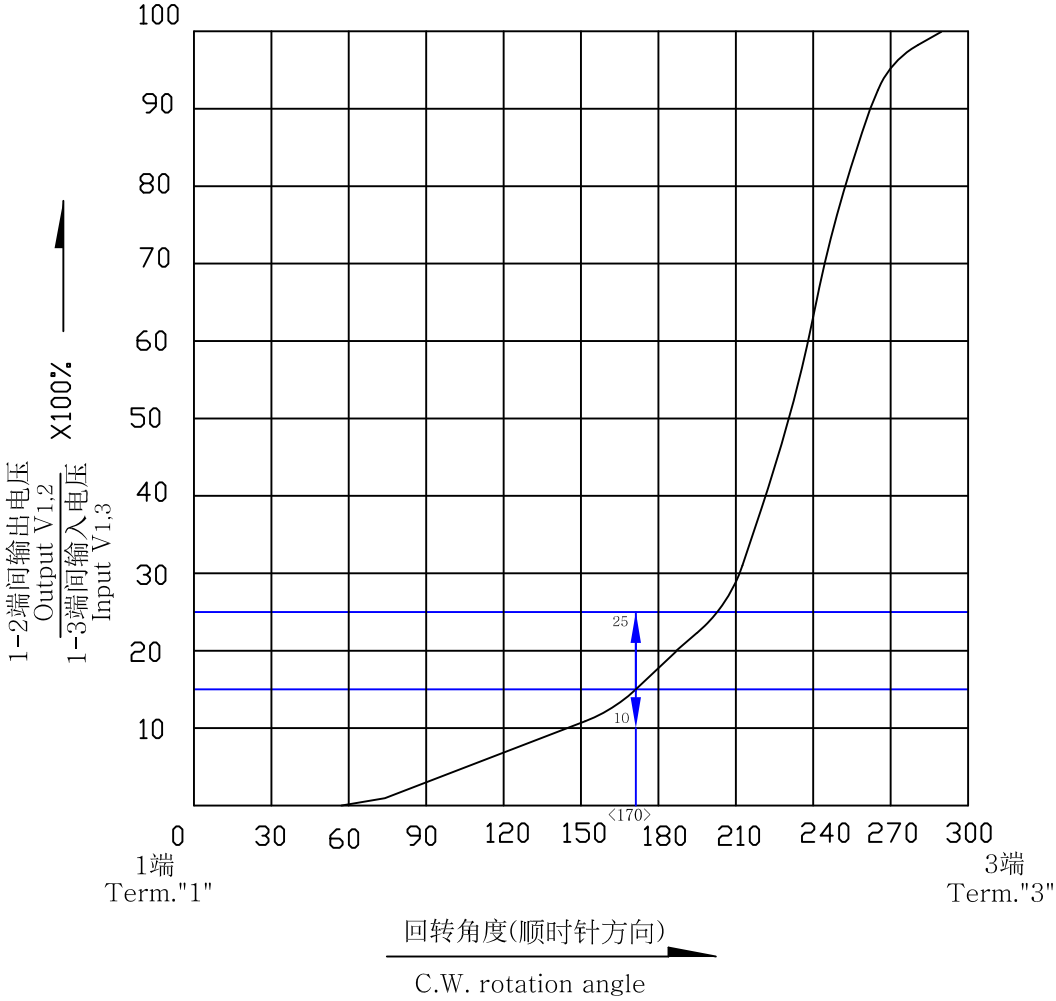
曲线变化特性: A(15A) TAPER A(15A)
