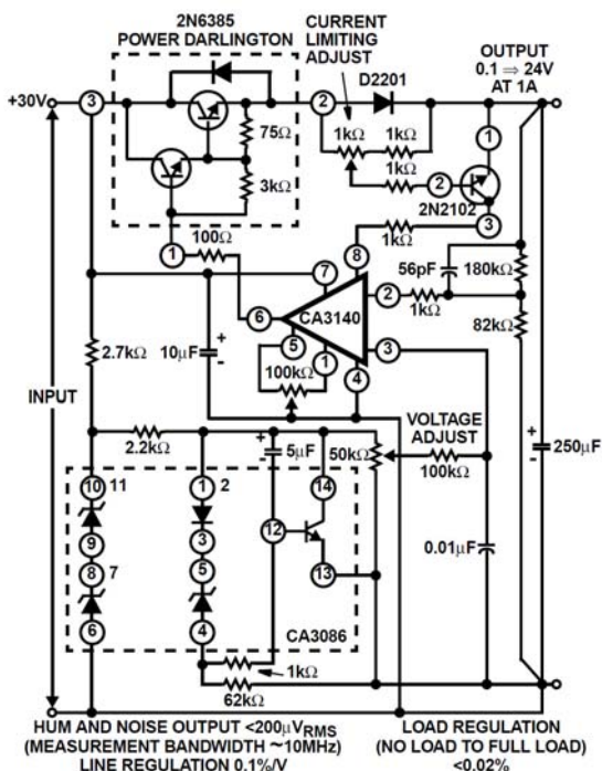
稳压电源电路
