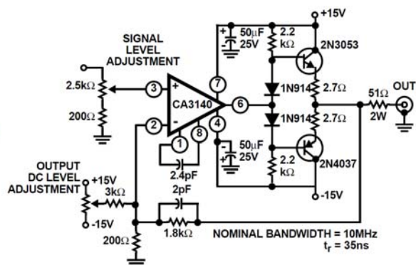
宽带输出放大器
