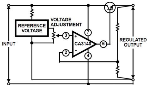
基本单电源电压调节器
