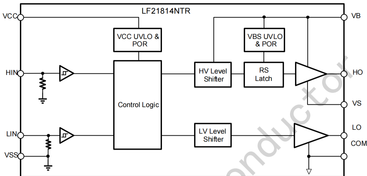
图7-1 LF21814NTR功能框图
