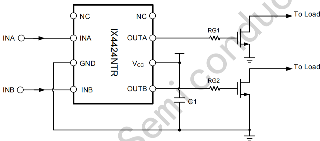
图 8-1 IX4424N 典型应用电路图
