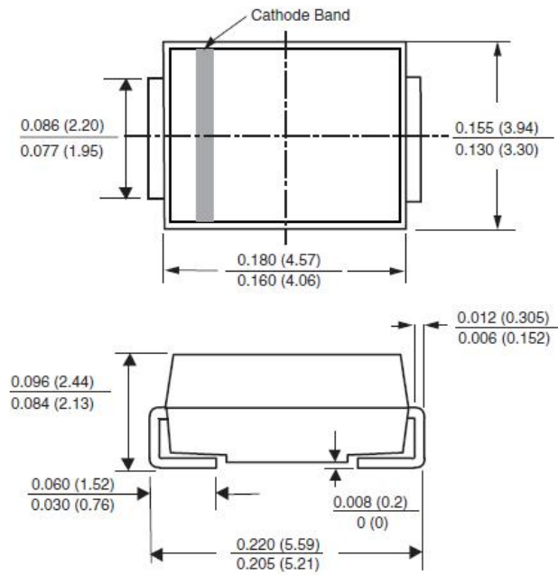
DO-214AA (SMB-J-Bend)
