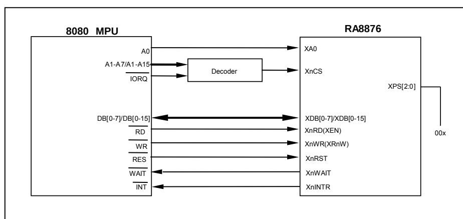
圖 7-1 : 8080 MPU Interface
