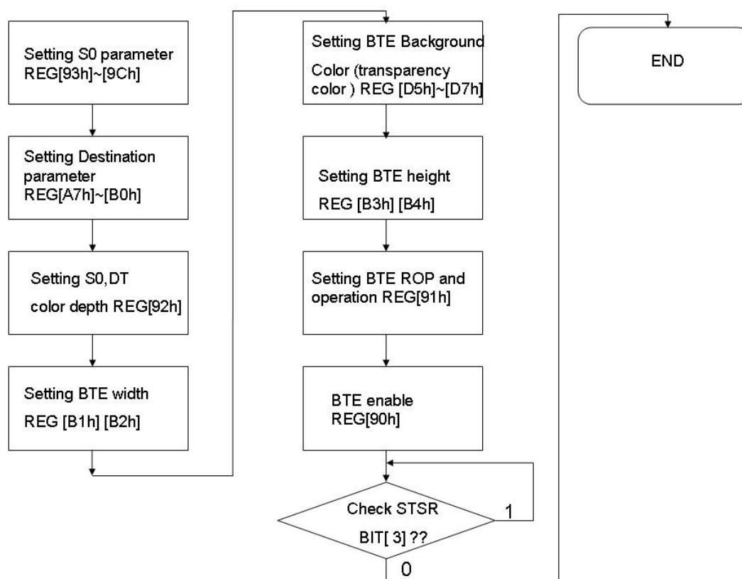
圖 13-12 : Flow Chart
