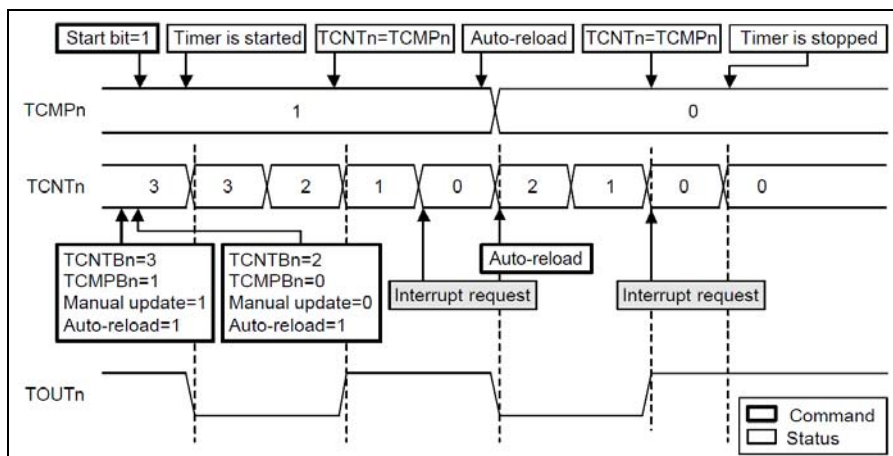
圖 15-2 : Timer Operations
