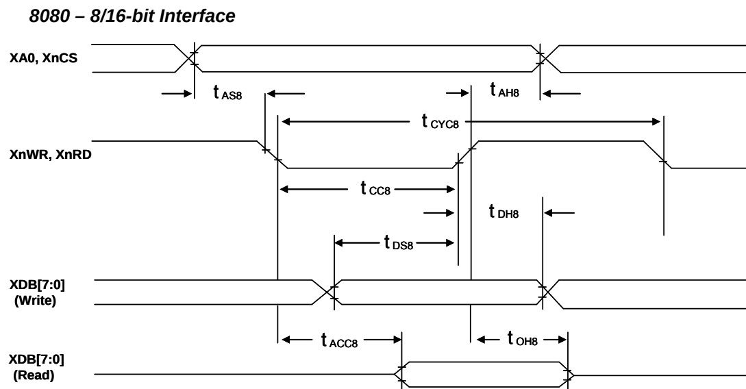
圖 7-3 : 8080 Waveform
