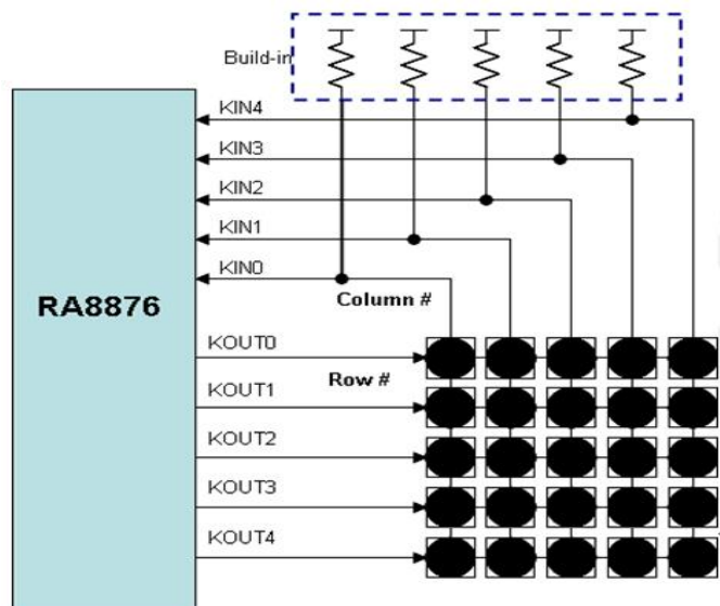
圖 17-1 : Key-Pad Application
