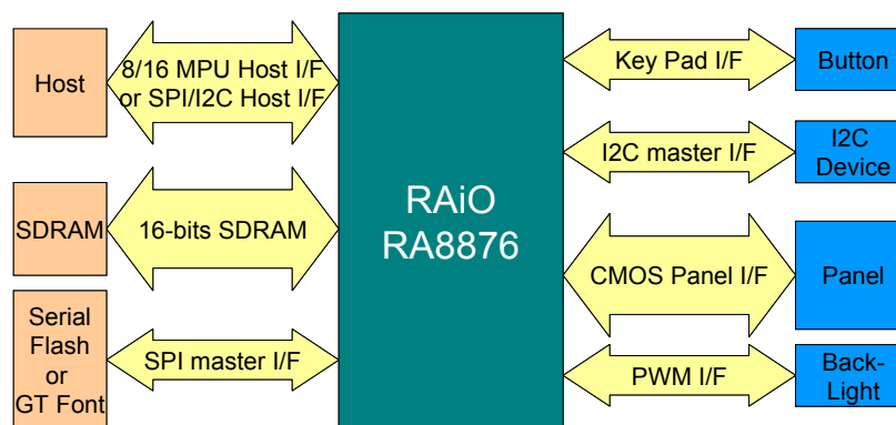
圖 1-1 : System Diagram
