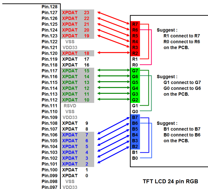
Figure 10-2 : RA8876 色深 18bit 脚位与 LCD 螢幕脚位对应
