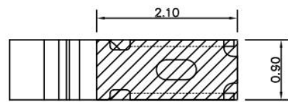
焊盘尺寸 尺寸公差 ±0.05
