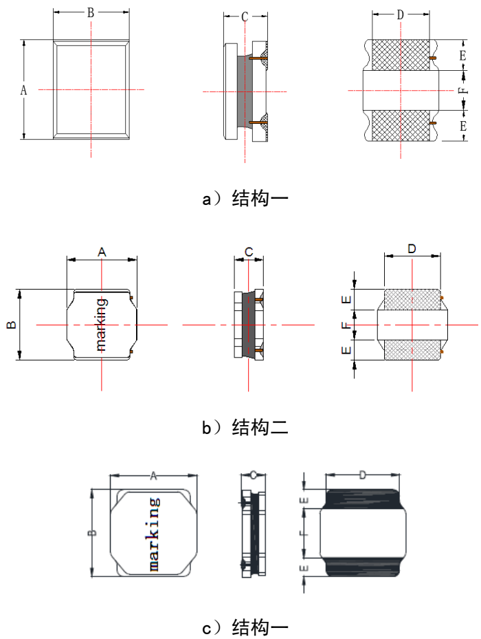
图 1 外形结构
