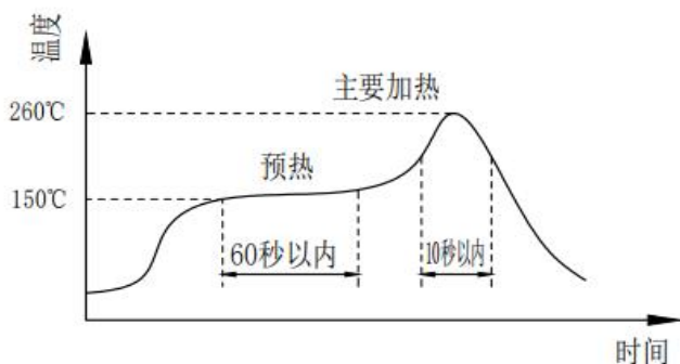
图 4.回流焊接
