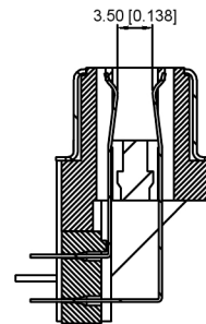
剖面 A-A
