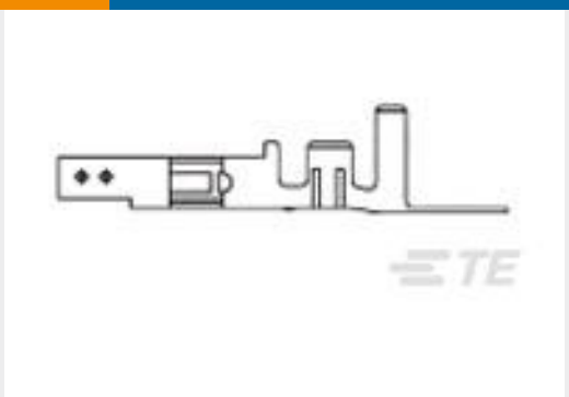
TE Part #794958-2 VAL-U-LOK SKT BR AU 22-26AWG
