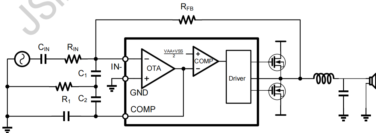
图 8-3 JSM2092S典型控制环路设计
