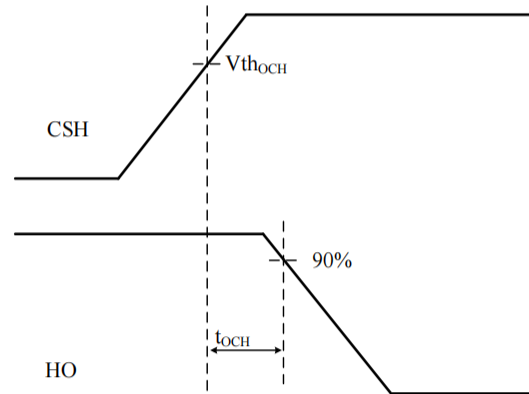
图 6-4 V_{CSH} > V_{thOCH} 至输出关断的波形及参数定义
