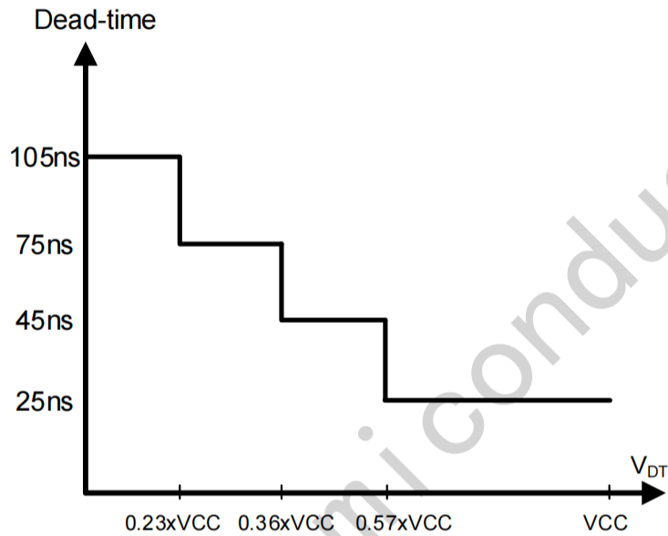
图 8-6 JSM2092S中死区时间与 V_{DT} 的关系
