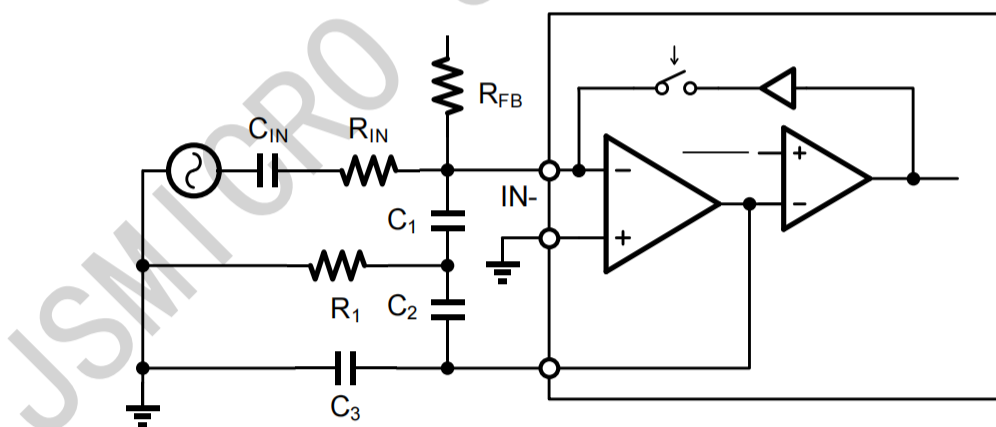
图 8-4 JSM2092S “咔哒”噪声消除机制
