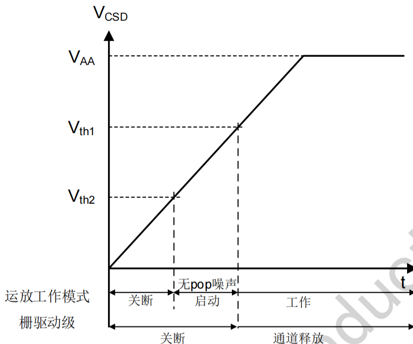
图 8-5 JSM2092S V_{CSD} 和运算放大器的工作模式
