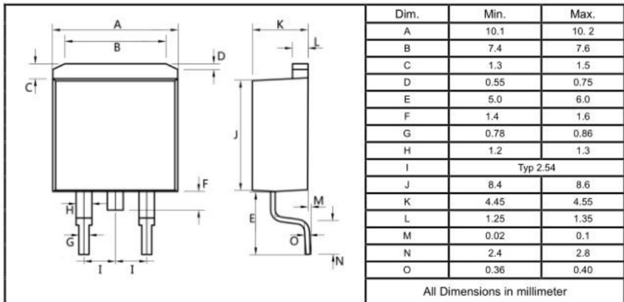
TO-263
