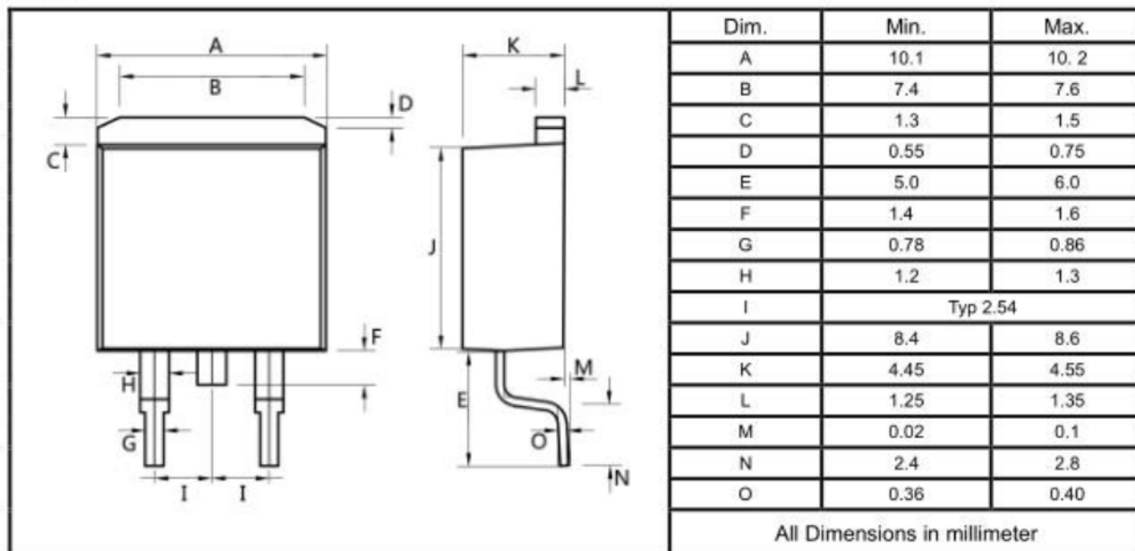
TO-263
