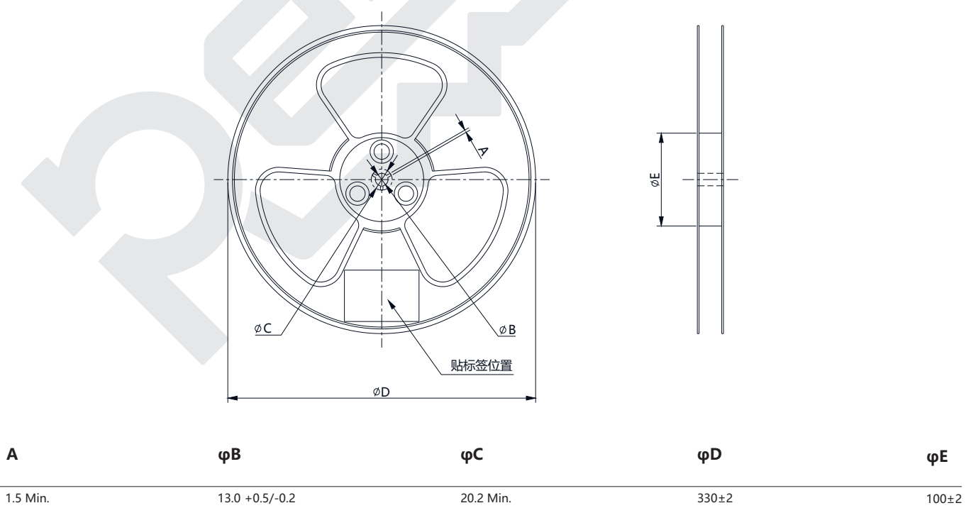
卡盘尺寸图
