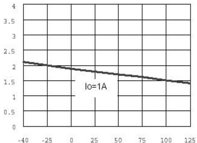
图4 下降电压
