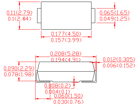
SMA(DO-214AC)
