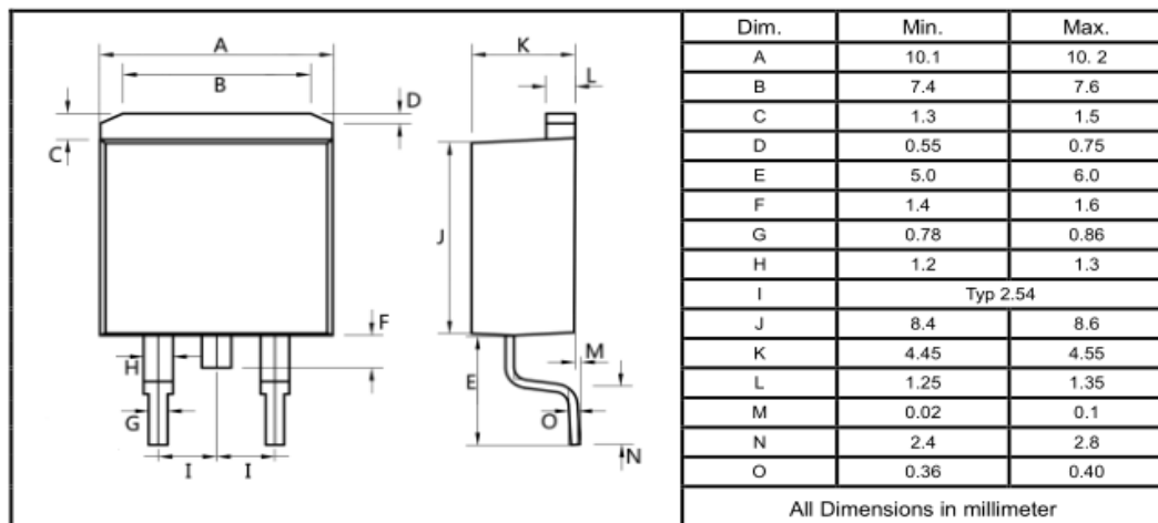
TO-263
