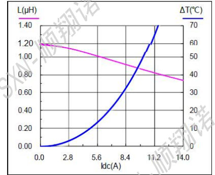
SMMS0530-1R2M
