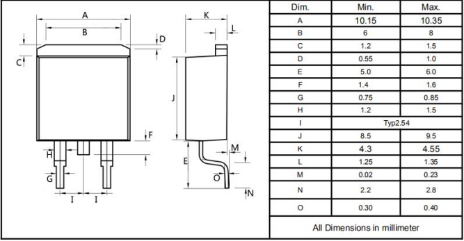
TO-263
