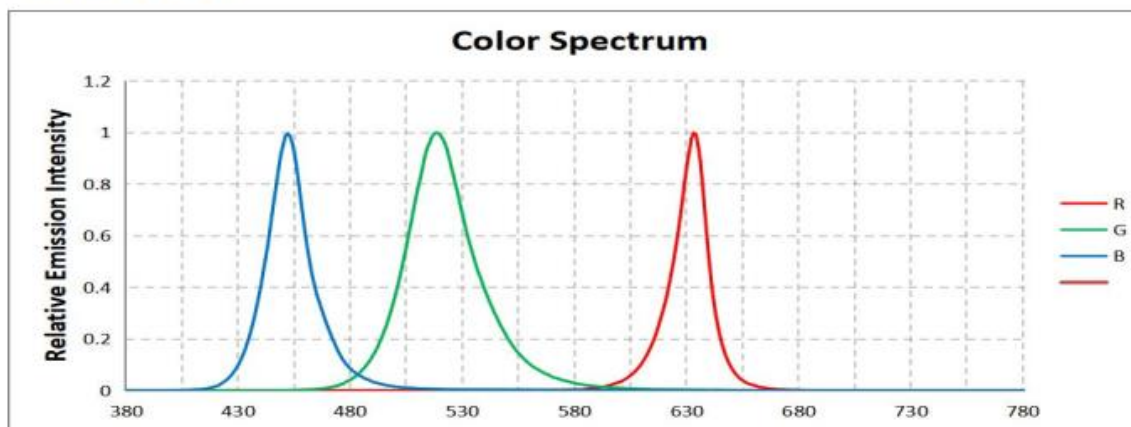
光谱图, Ta=25°C
