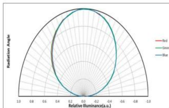
角度图, Ta=25°C
