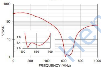
VSWR
