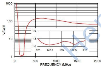
VSWR
