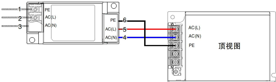
图 1: EMC 更高要求推荐电路
