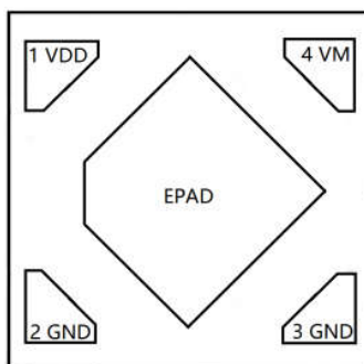
图 1 DFN1*1-4L引脚定义图
