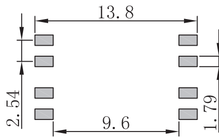
焊盘尺寸/Pad Size
