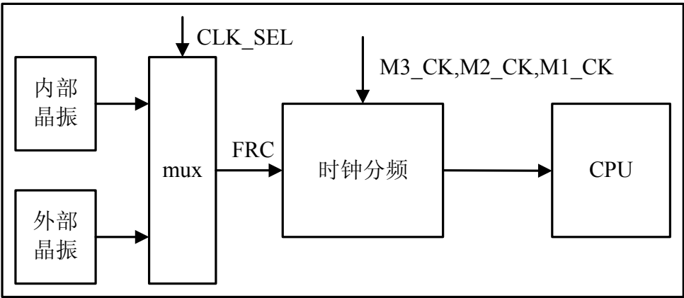
图 2-7 CPU 指令周期时钟示意图
