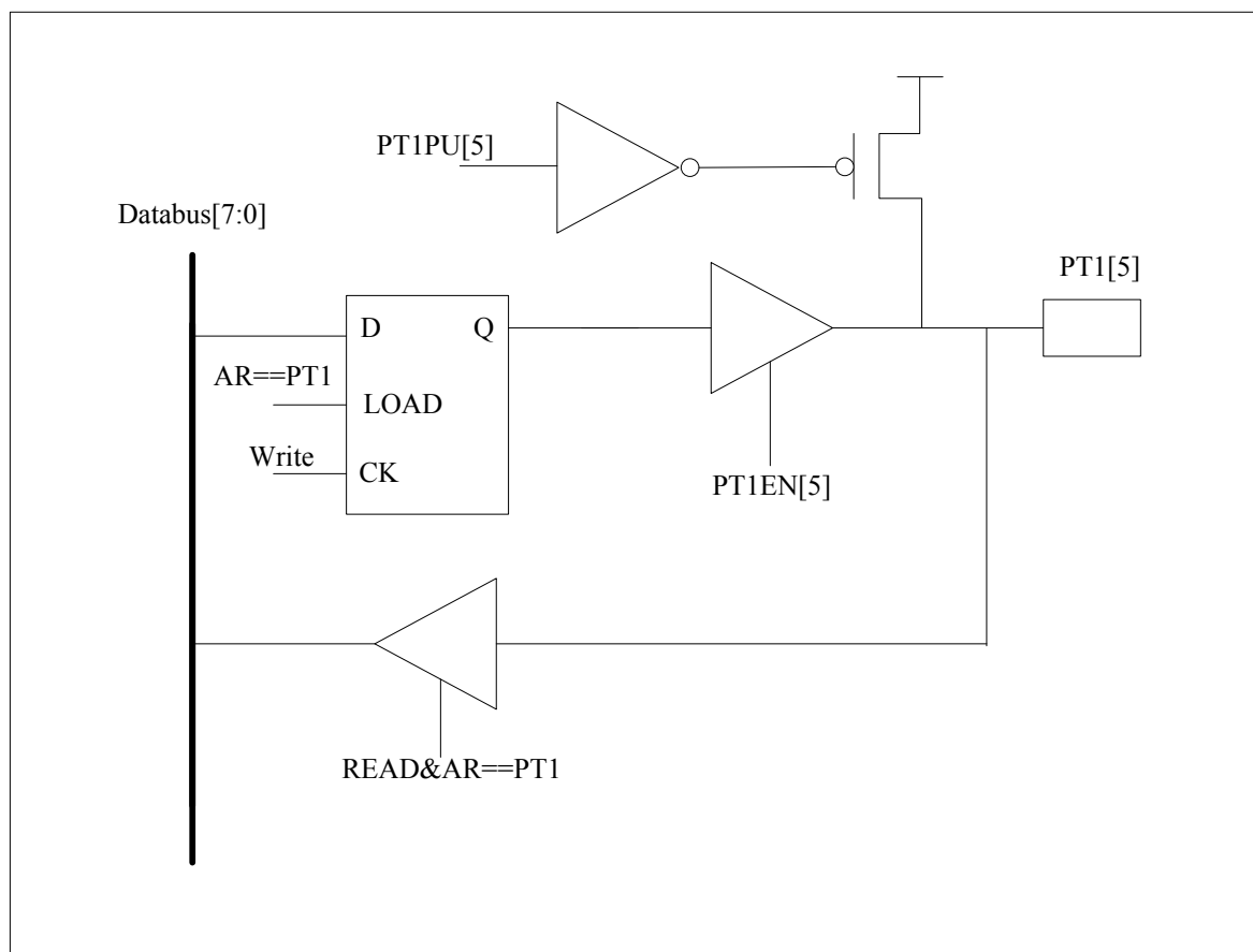
图 2-15 PT1[5] 功能框图
