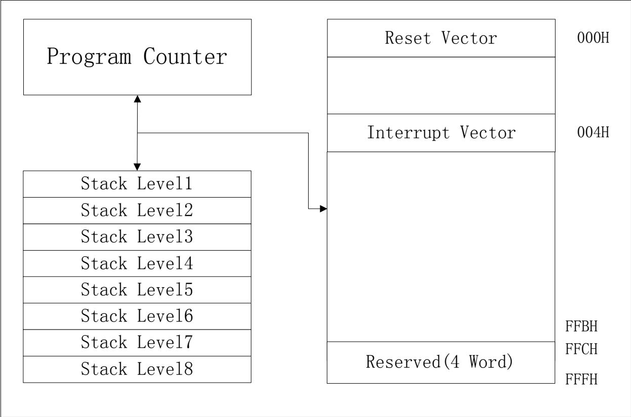
图 2-2 程序存储器
