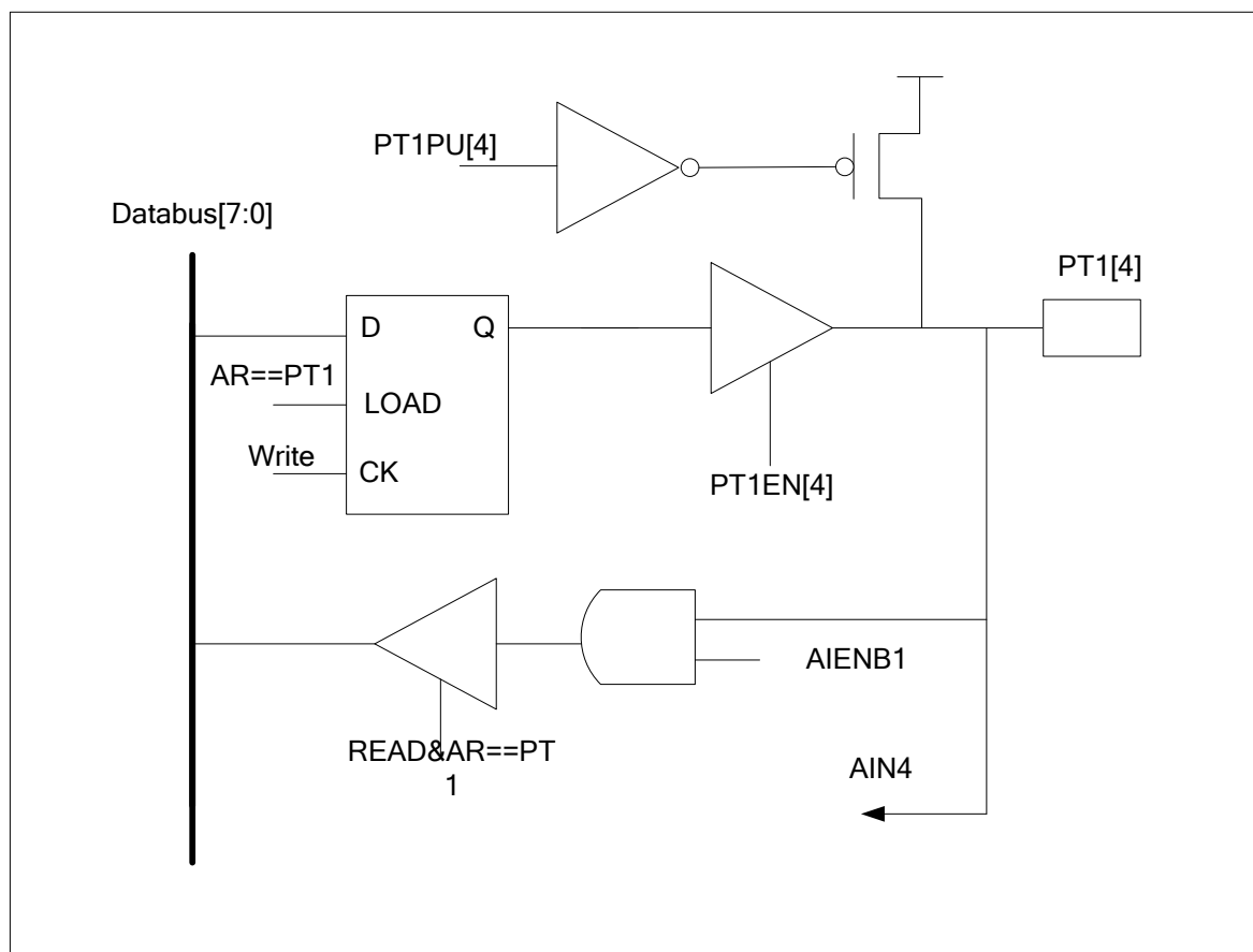
图 2-14 PT1[4] 功能框图
