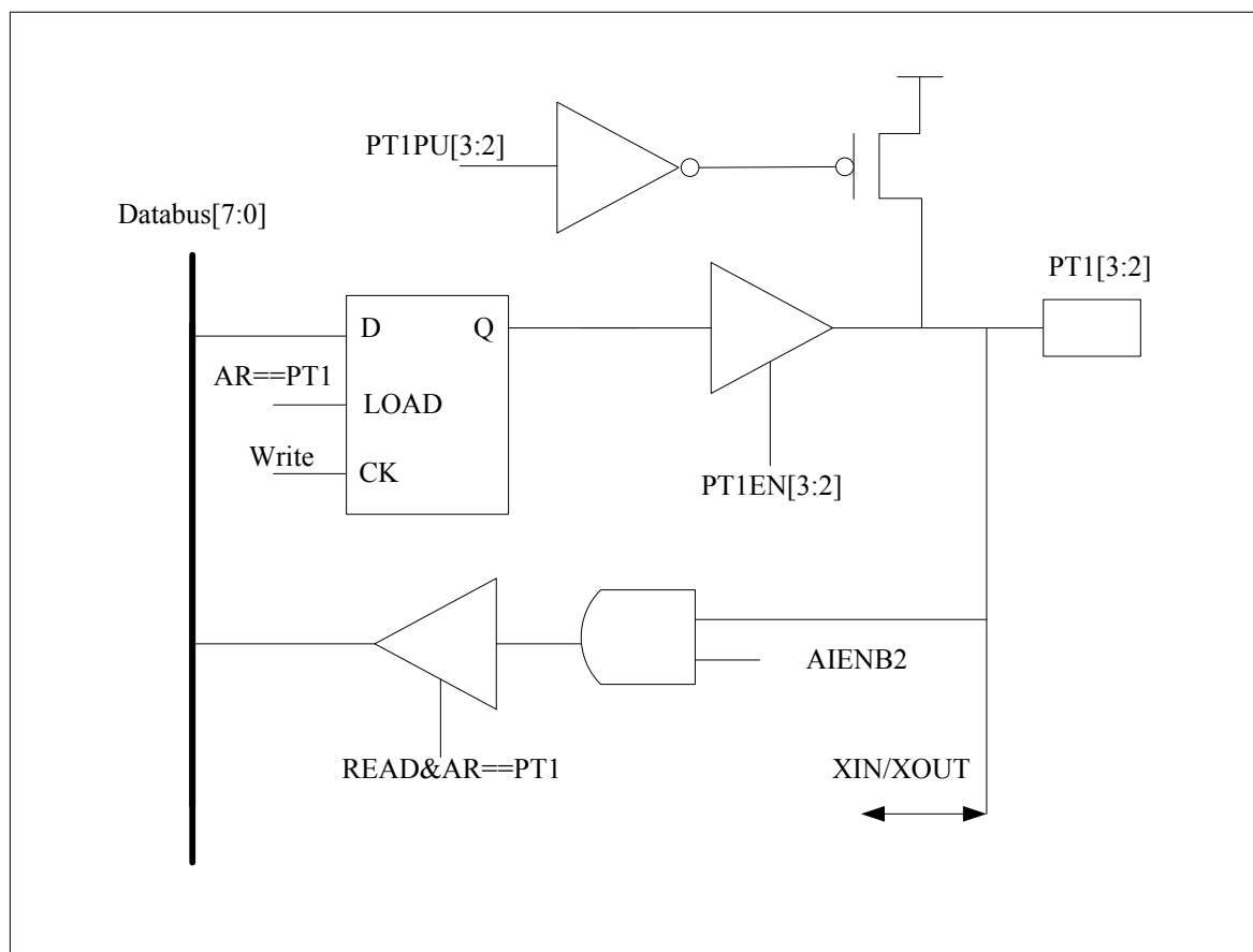
图 2-13 PT1[3:2] 功能框图
