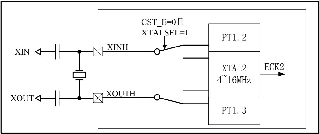
图 2-6 外部振荡器 2
