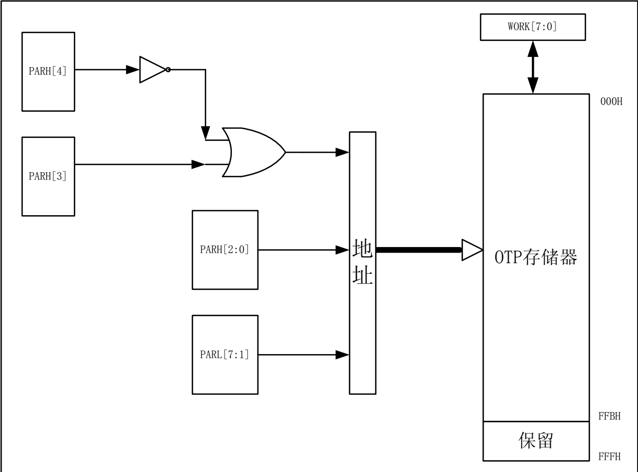
图 3-25 在线烧录地址寻址
