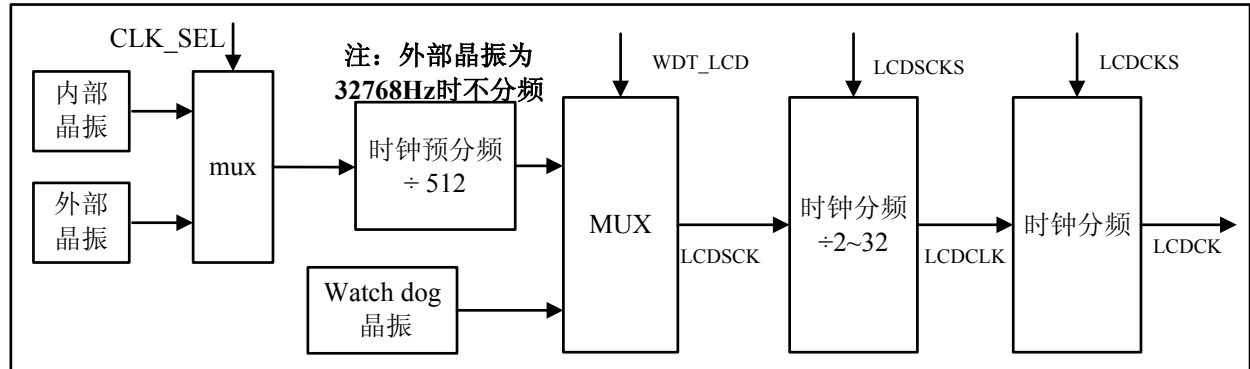
图 2-10 LCD 帧频时钟选择
