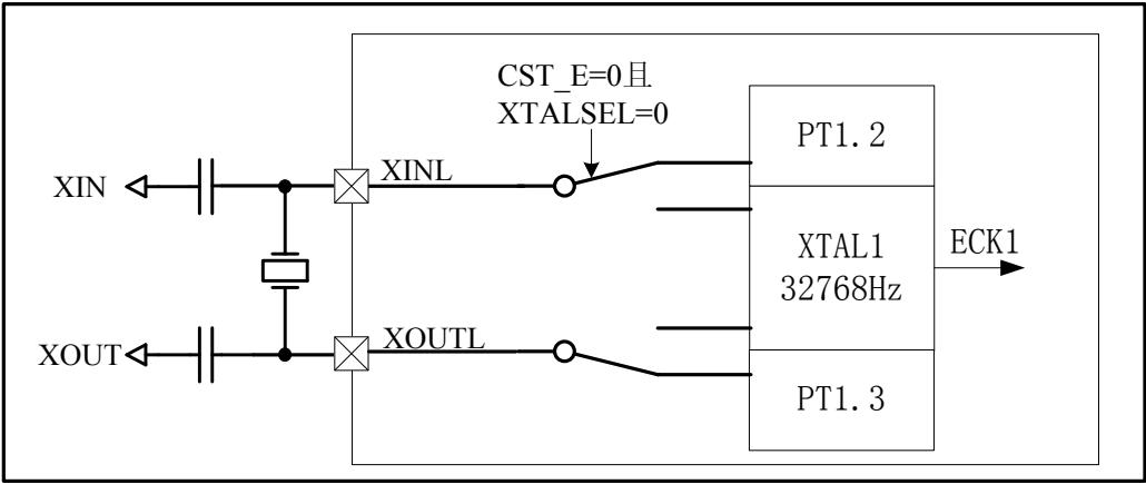
图 2-5 外部振荡器 1
