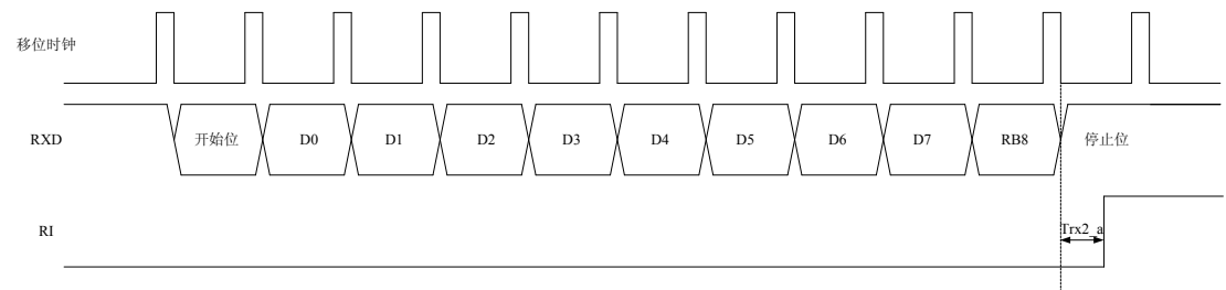
图 3-23 UART 模式 2 接收数据波形
