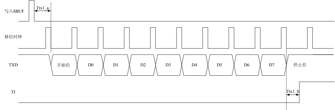
图 3-20 UART 模式 1 发送数据波形
