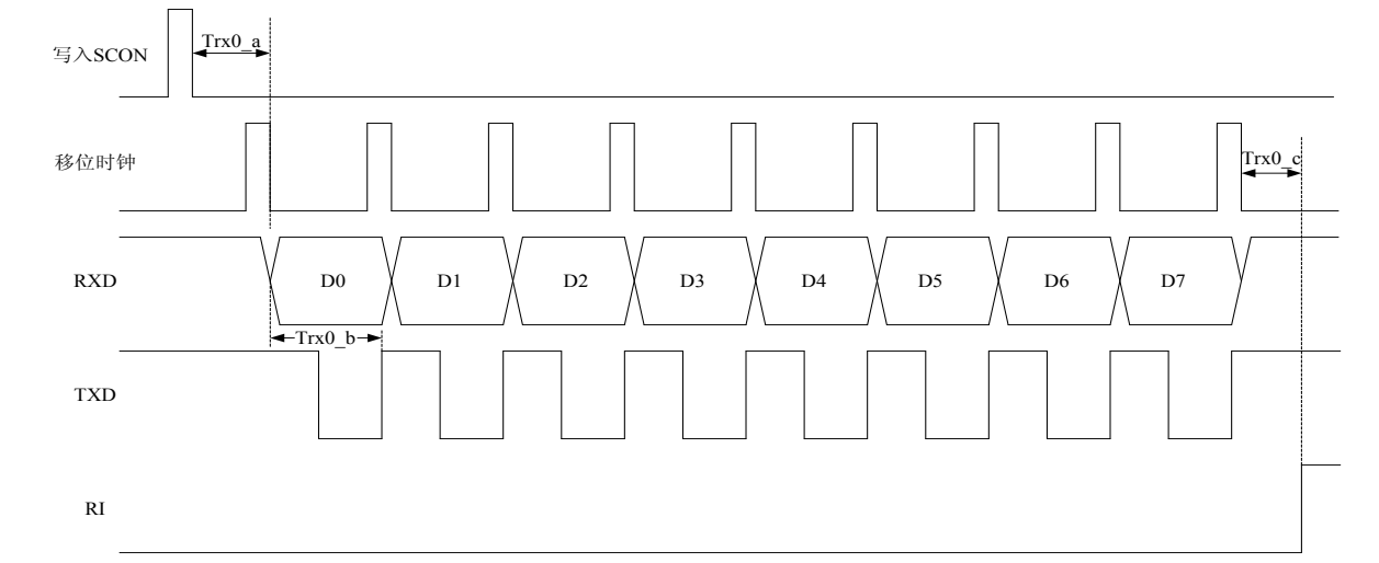
图 3-19 模式 0 接收数据波形
