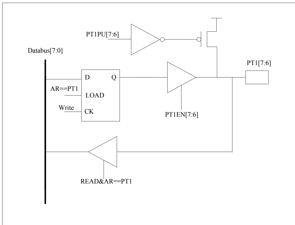
图 2-16 PT1[7:6] 功能框图
