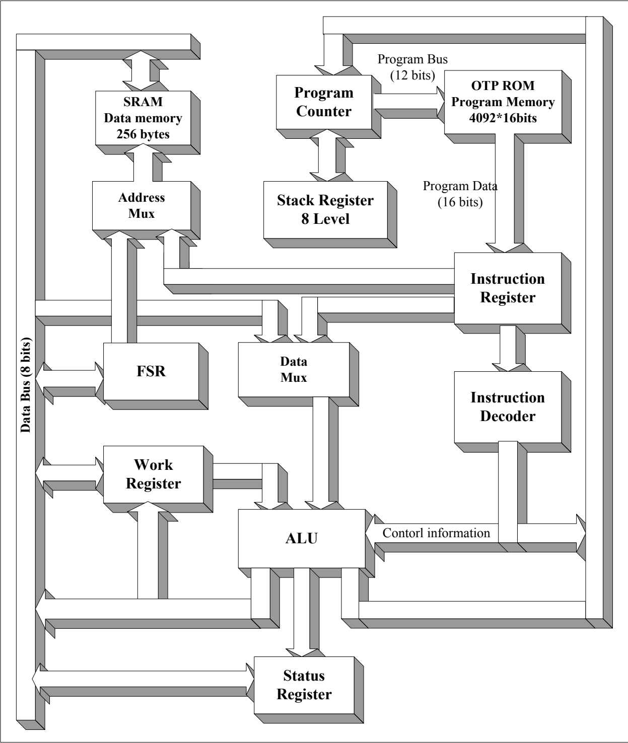
图 2-1 CSU8RP1186B CPU 核的功能模块图
