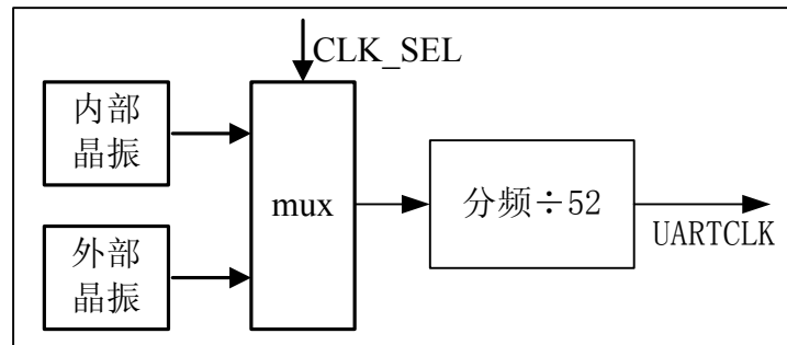
图 2-11 UART 时钟分频示意图
