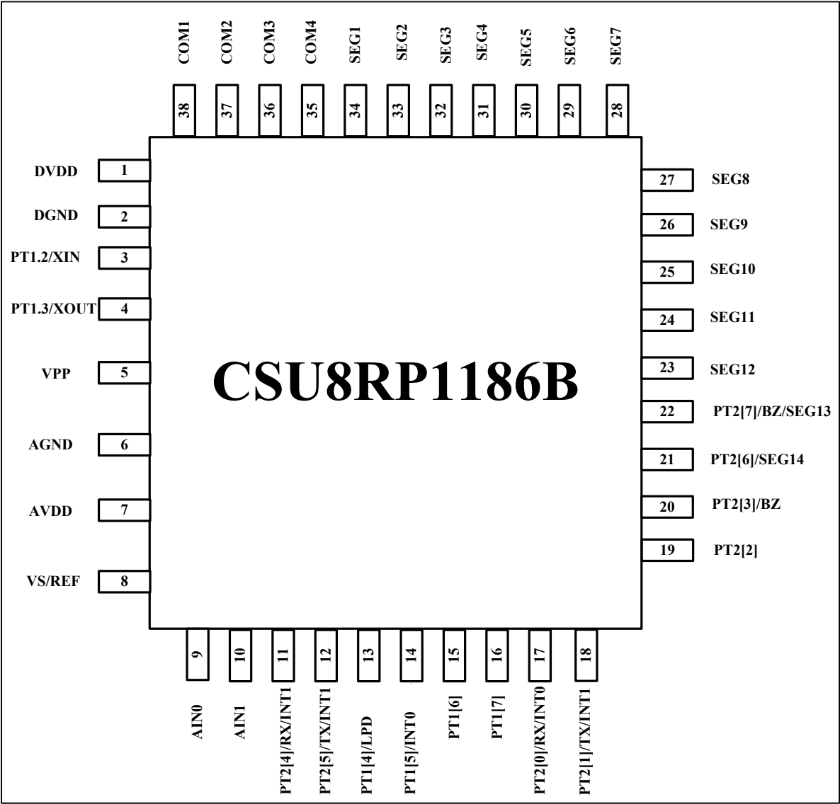
图 1-1 功能引脚图
