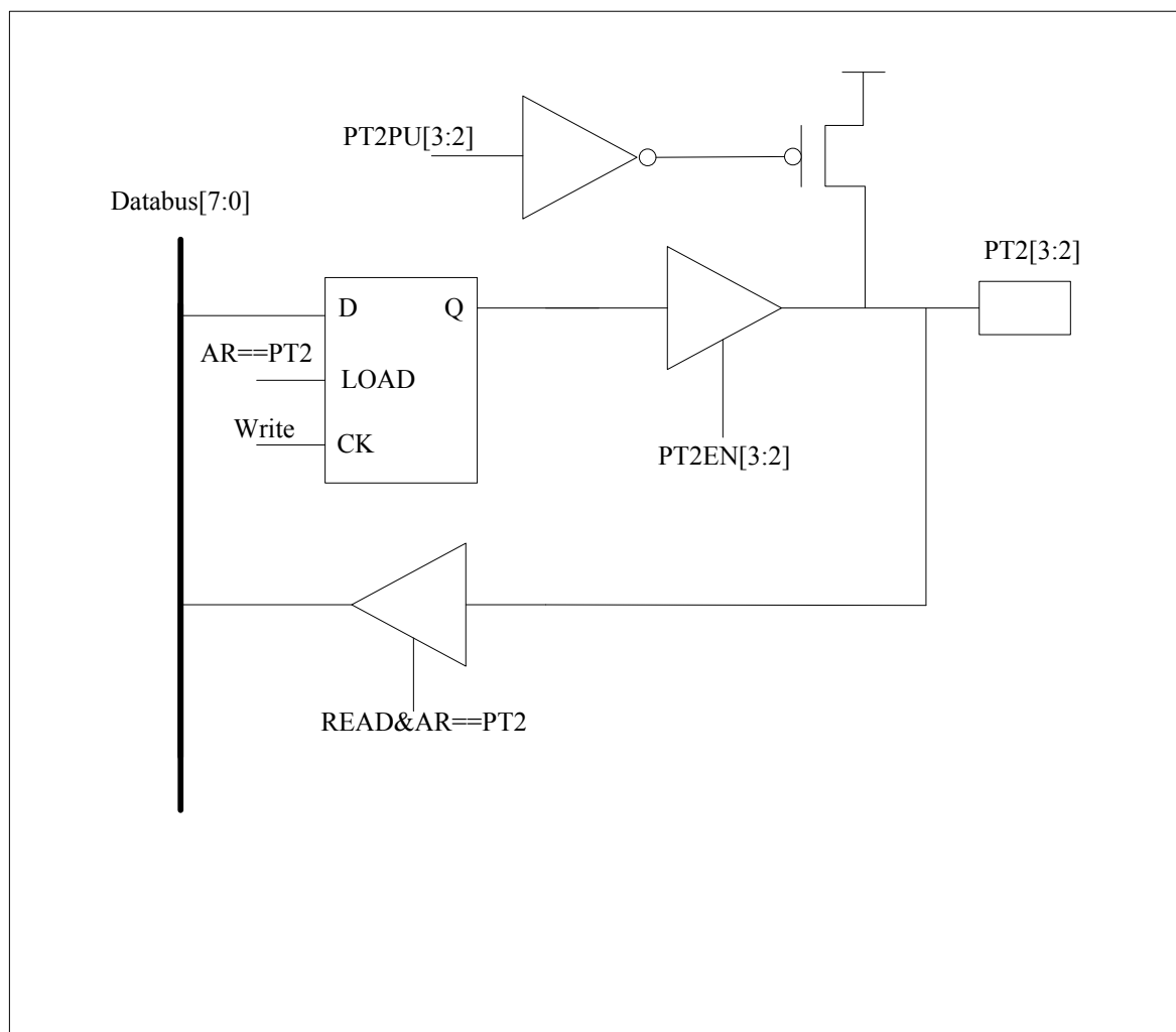
图 2-18 PT2[6:2] 功能框图
