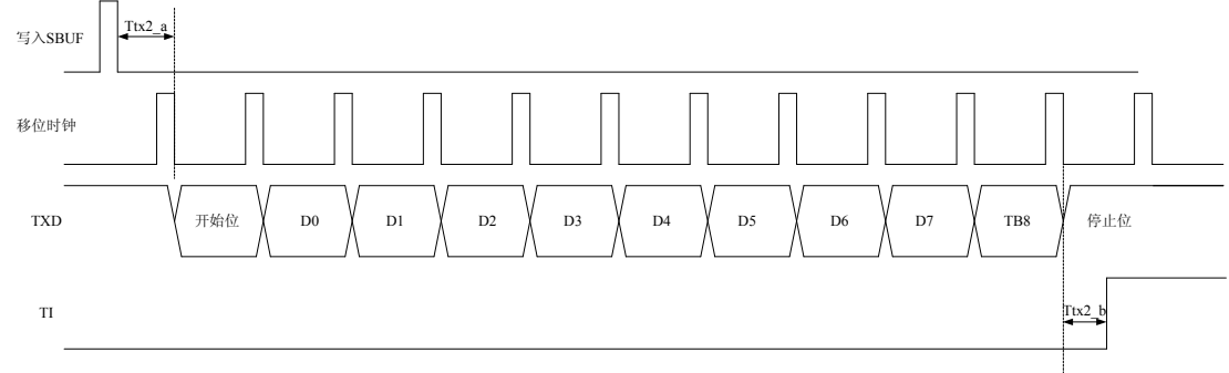
图 3-22 UART 模式 2 发送数据波形
