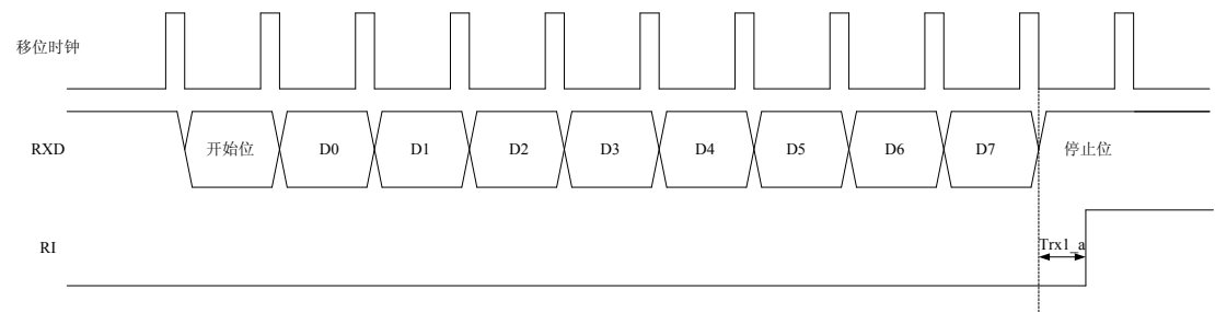
图 3-21 UART 模式 1 接收数据波形
