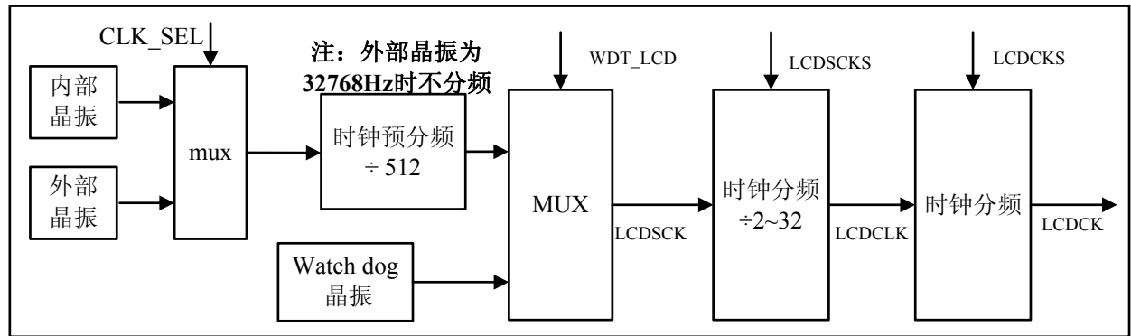
图 3-7 LCD 帧频时钟选择
