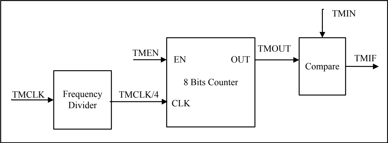
图 2-12 定时模块的功能框图
