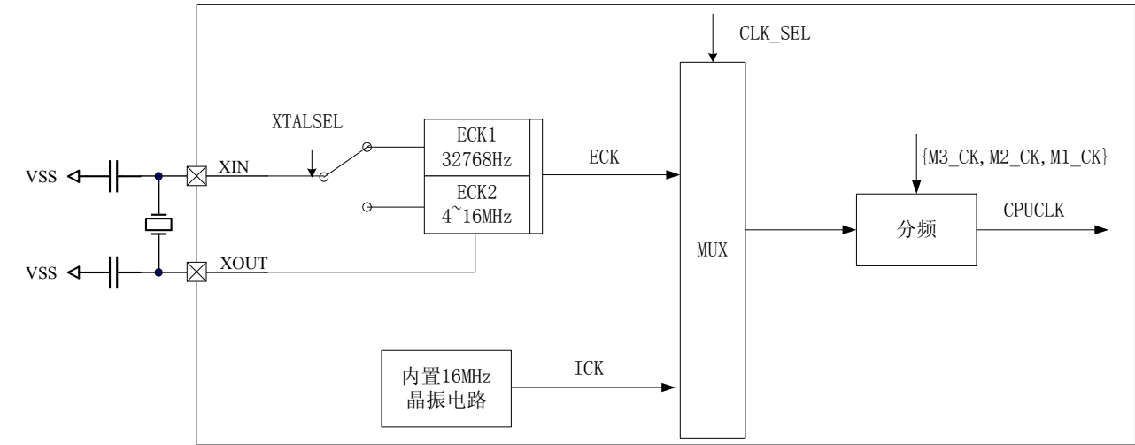
图 2-4 CSU8RP1186B 振荡器状态框图
