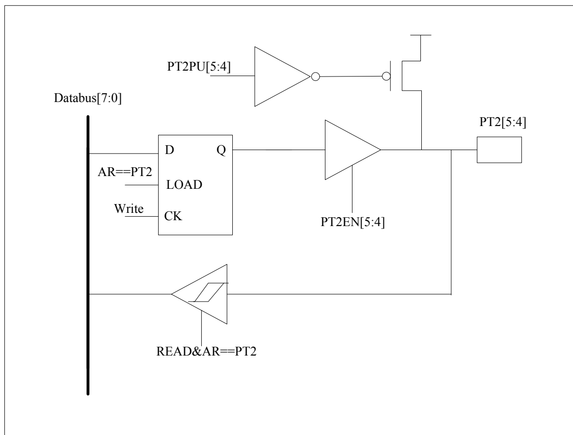
图 2-19 PT2[5:4]功能框图
