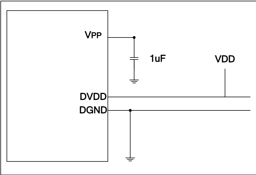
图 3-3 电荷泵外围电路示意图
