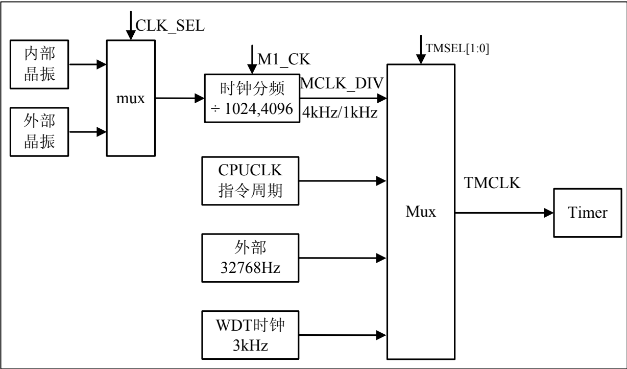
图 2-9 定时器时钟分频示意图
