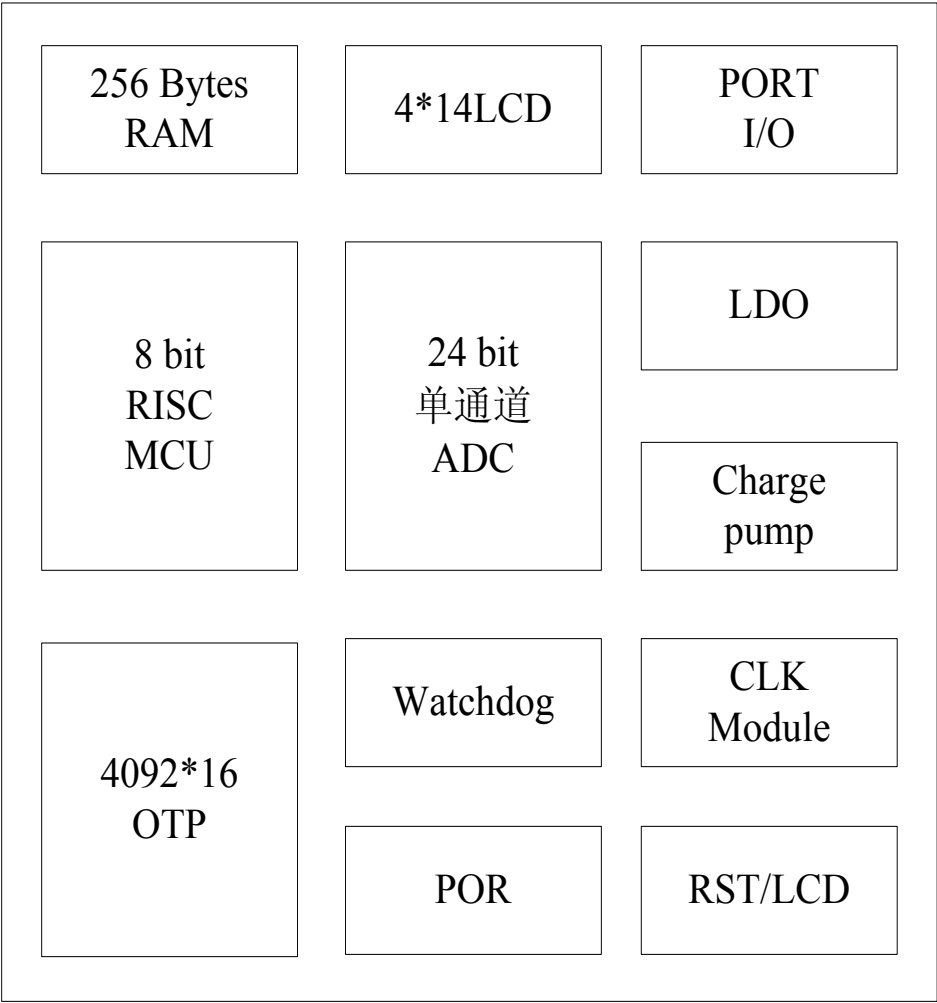
图 1-2 CSU8RP1186B 功能模块
