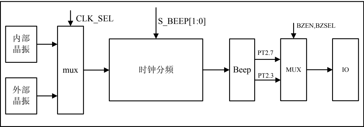
图 2-8 Beep 时钟选择示意图
