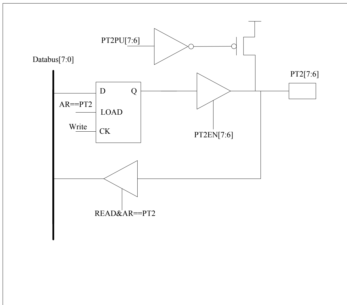
图 2-20 PT2[7:6] 功能框图
