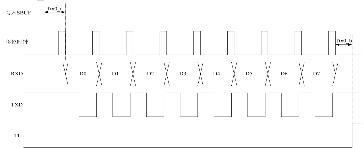
图 3-18 模式 0 发送数据波形
