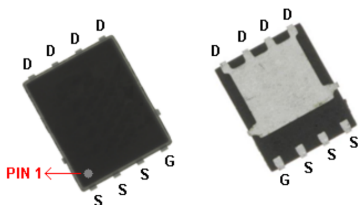
PowerDFN 5x6
