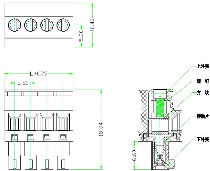
外形尺寸（Shape Dimension）
