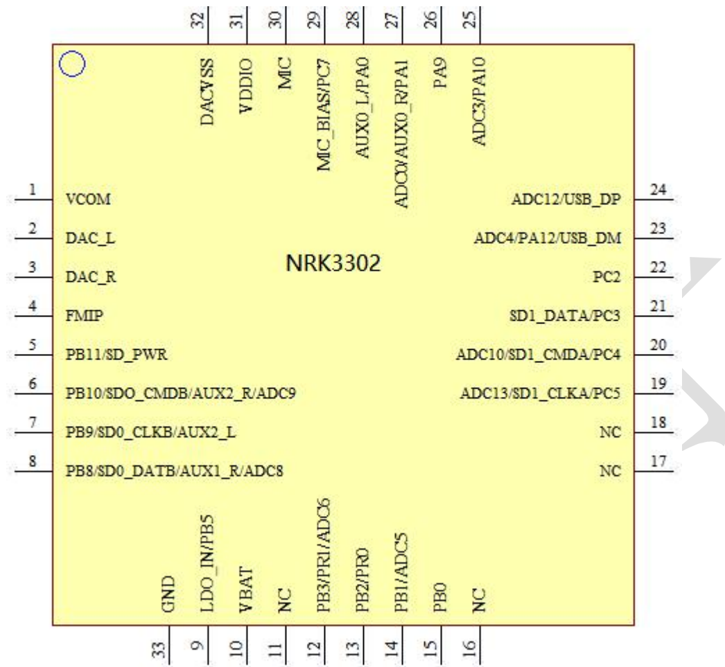
NRK3302引脚图
