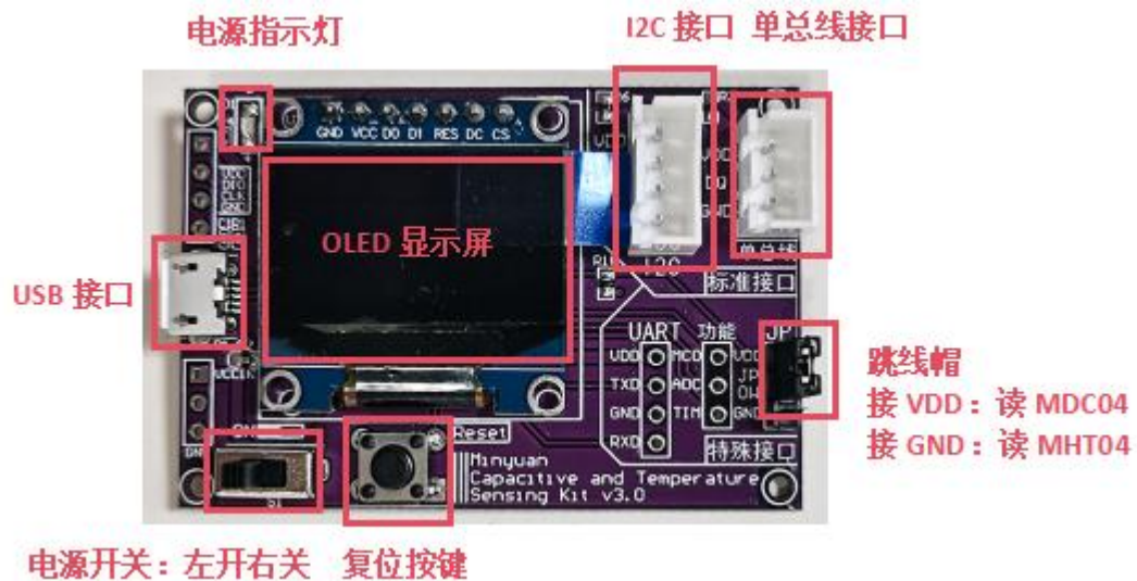
图2. MCSK主板构成
