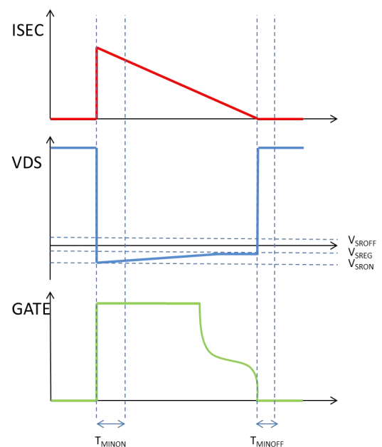
图二 同步芯片开启及关断时序
