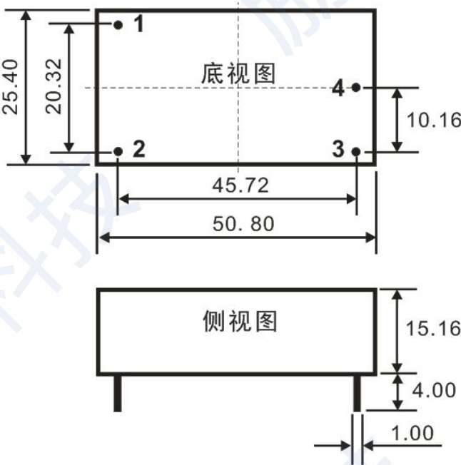
单位：mm 公差：±0.5mm
