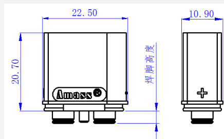
焊脚高度
