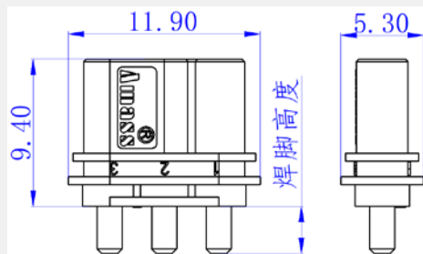
焊脚高度
