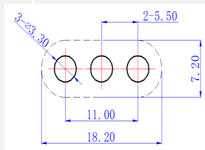
安装孔示意图
