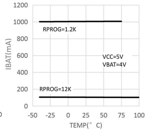
充电电流与环境温度的关系曲线
