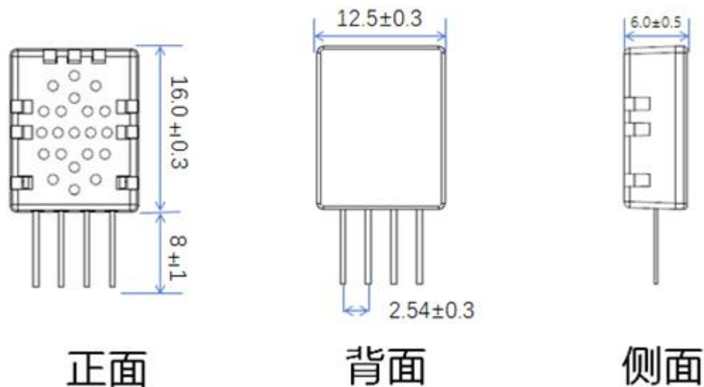
图 1: 模组结构图
