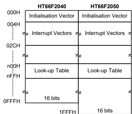
程序存储器结构
