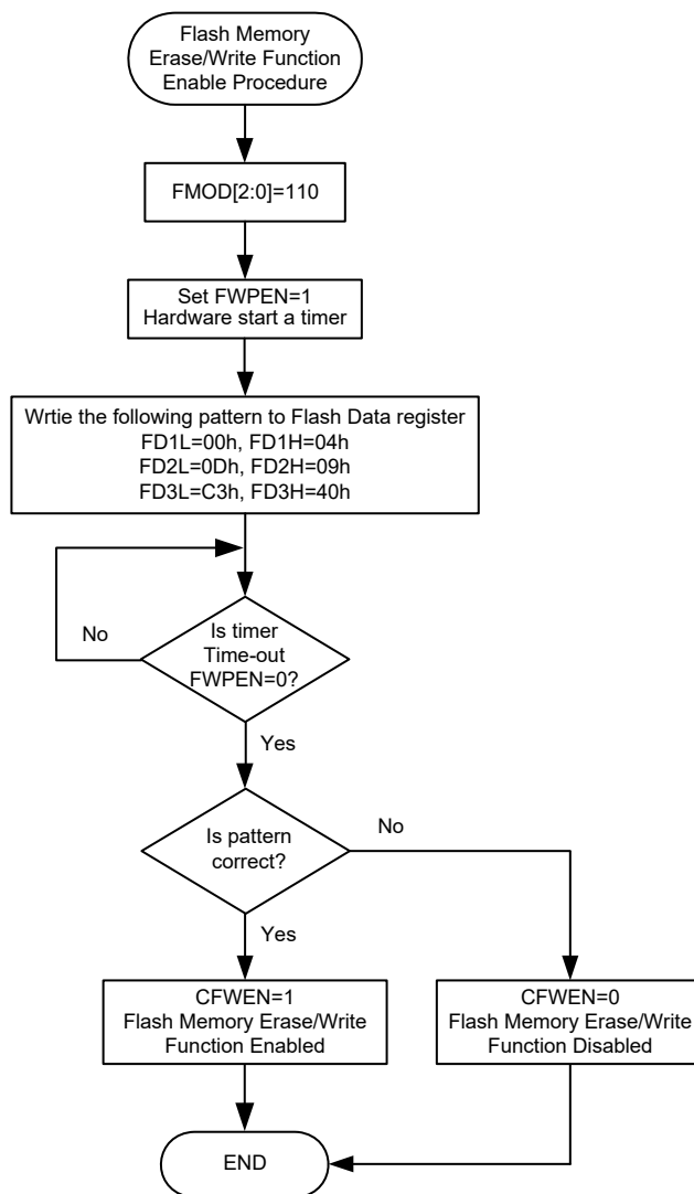
Flash 存储器擦 / 写使能步骤
