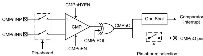
比较器 (n=0~1)
