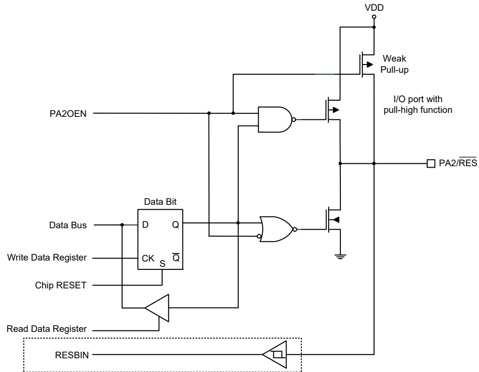
PA2 端口输出结构
