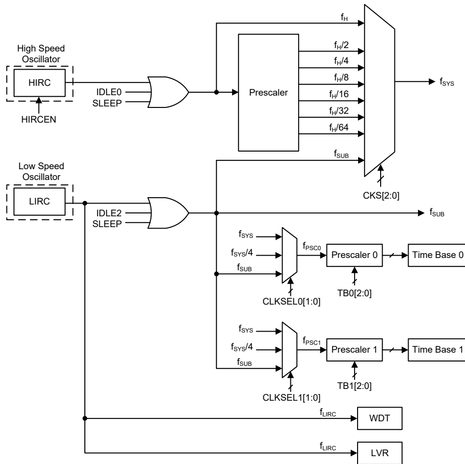
单片机时钟选项
