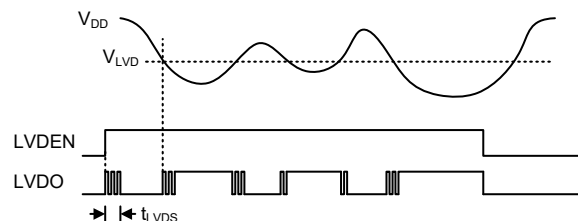
LVD 操作
