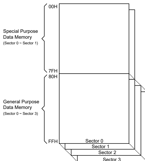
数据存储器结构
