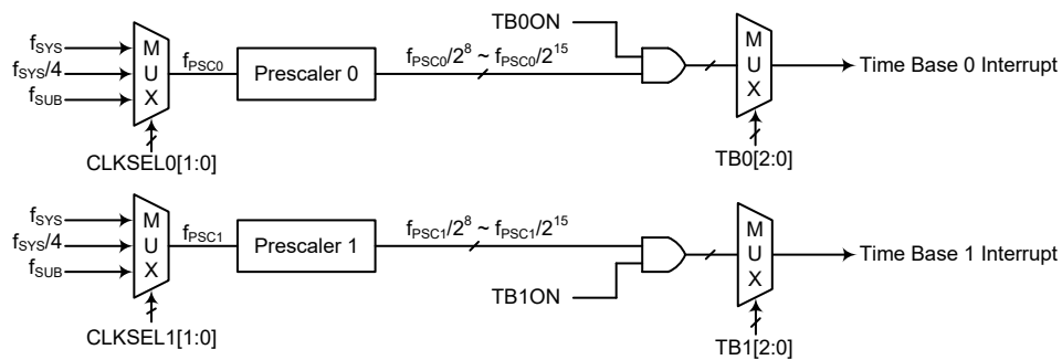
时基中断
