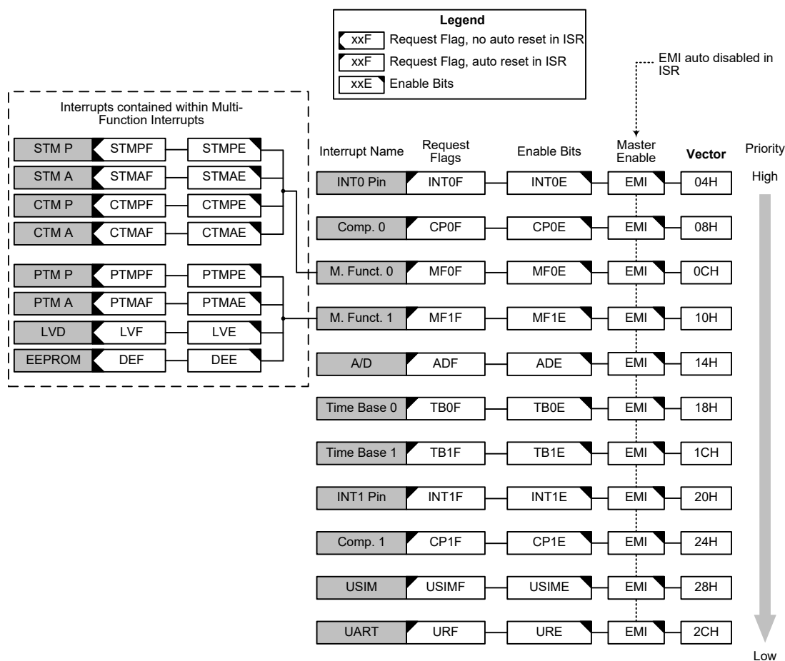
中断结构
